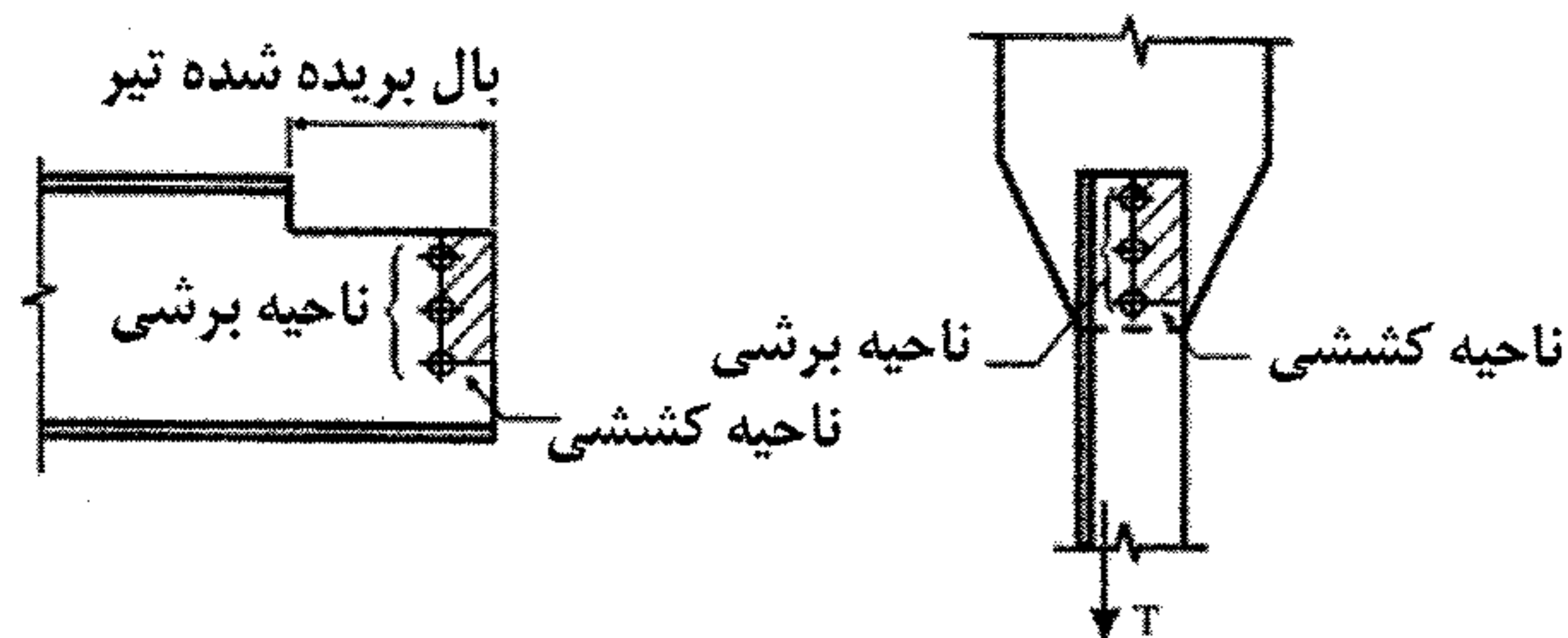
شکل ۱۰-۲-۹-۱۰-الف سطوح گسیختگی در برش قالبی
