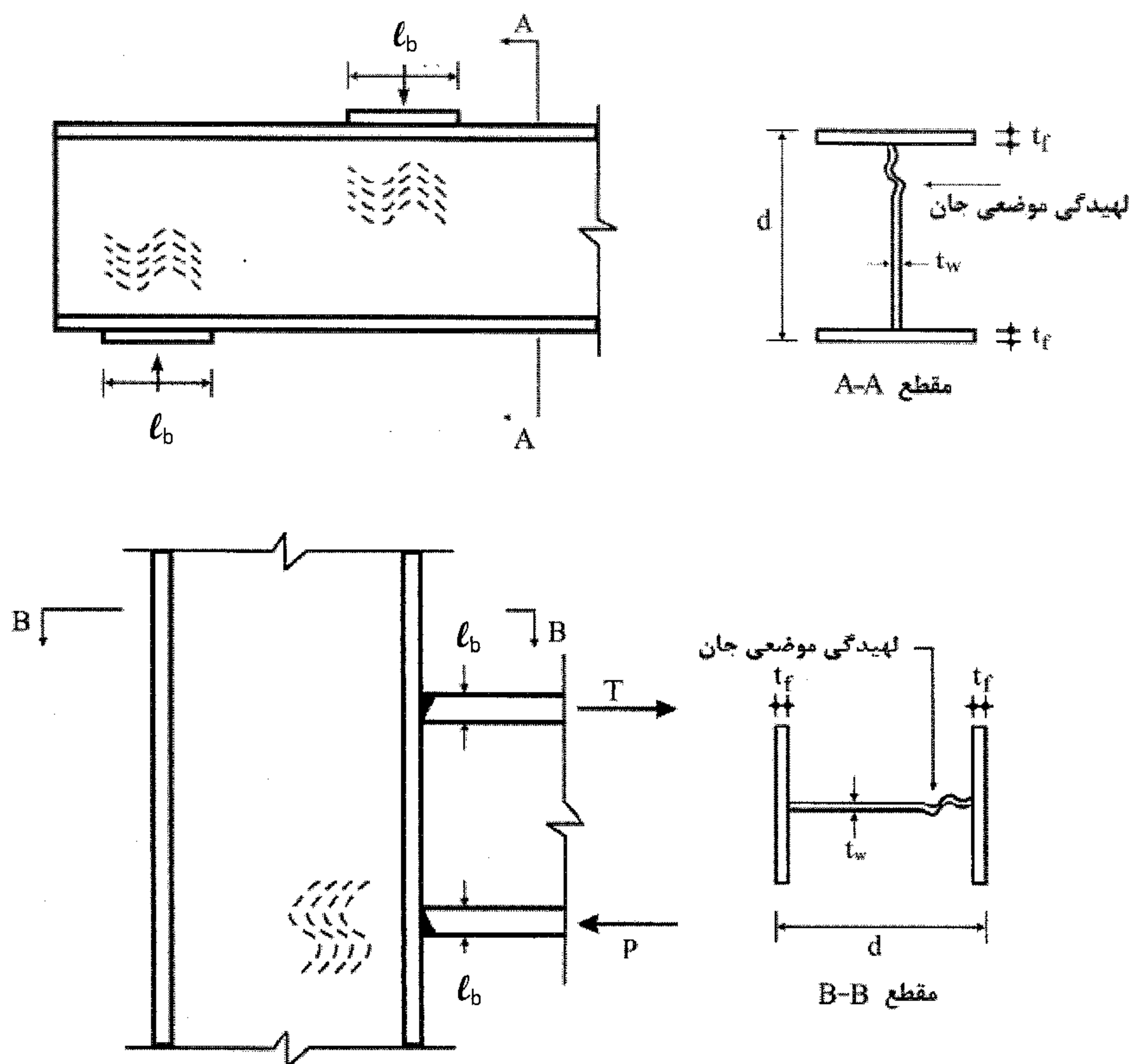
شکل ۱۸-۹-۲-۱۰ لپیدگی جان در مقابل نیروی متمرکز فشاری
