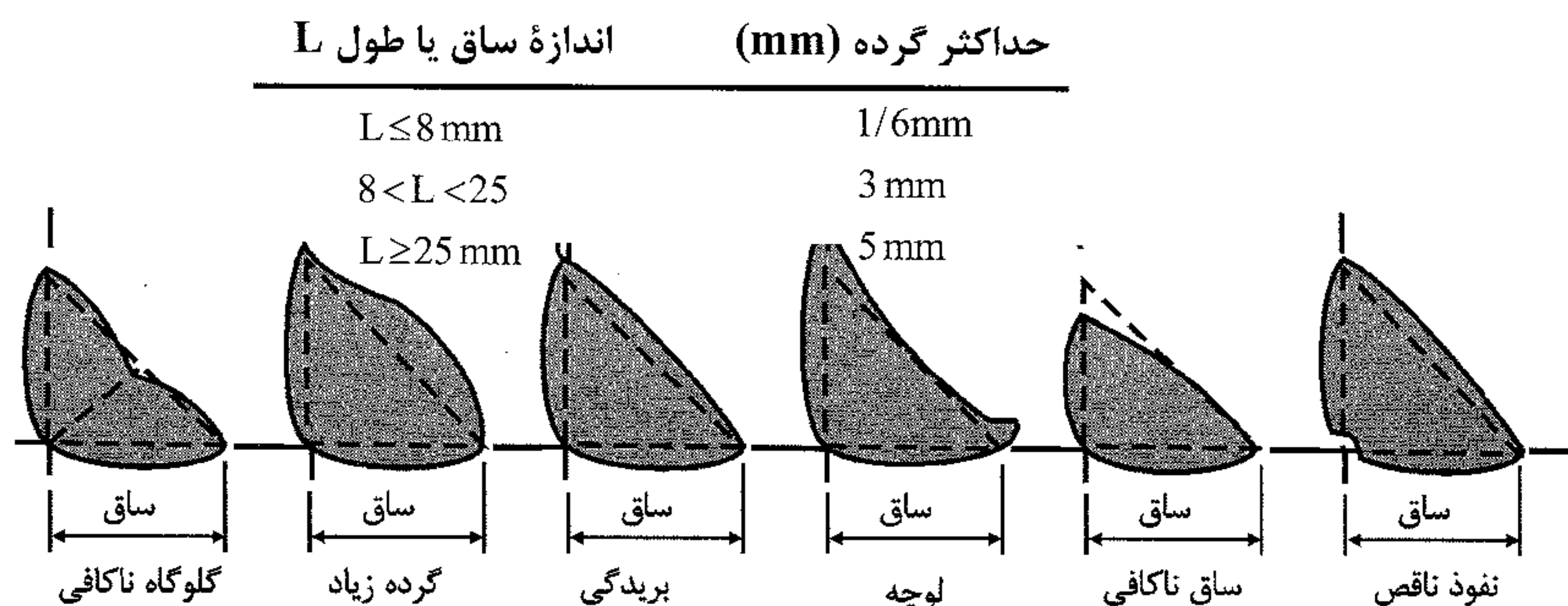
(پ) مقاطع غیر قابل پذیرش جوش گوشه
