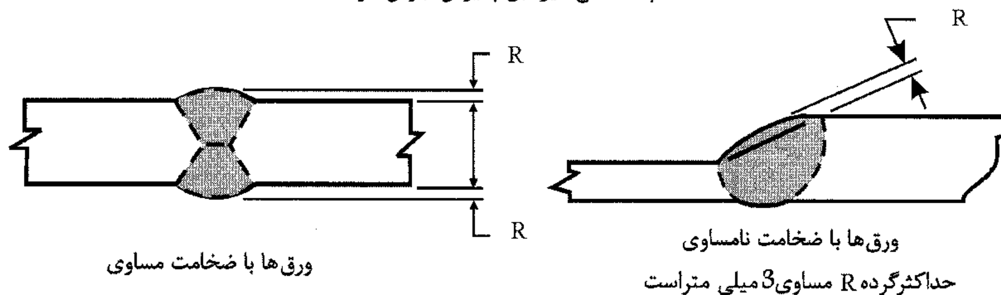
(ت) مقاطع قابل پذیرش جوش های شیار
