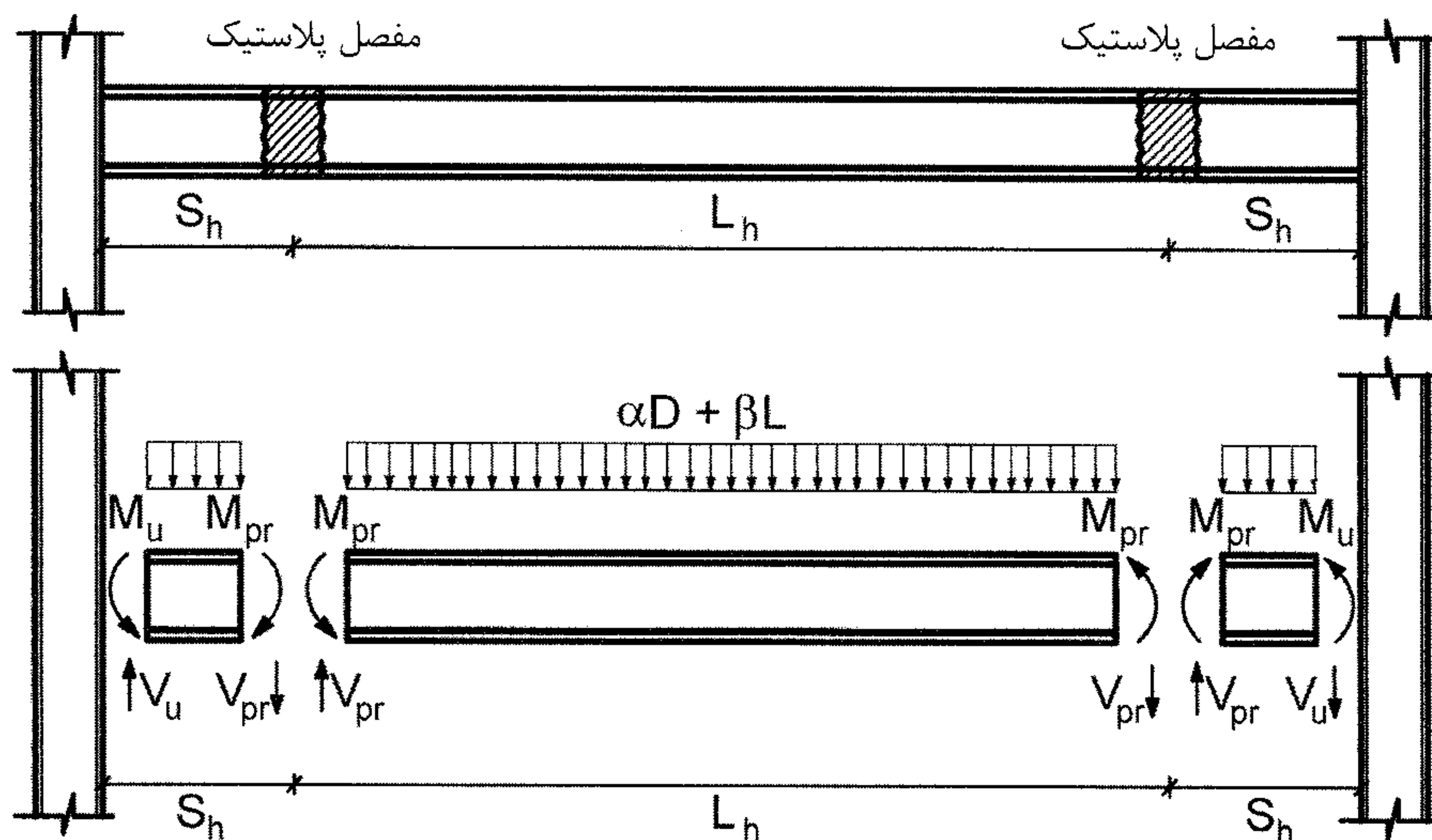
شکل ۳-۱۰-۸-۱ نمودار پیکره آزاد تیرهای باربر جانبی
