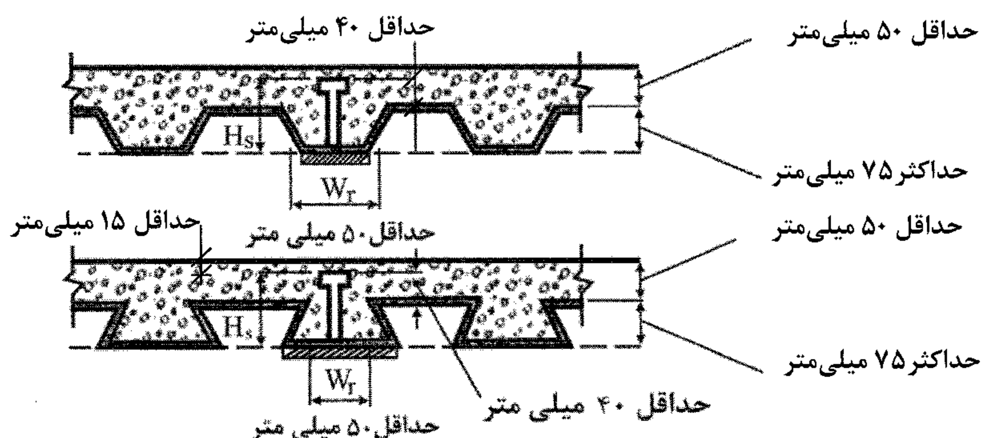
شکل ۲-۱۰-۸-۴ ملاحظات و محدودیت‌های ورق‌های فولادی شکل داده شده
