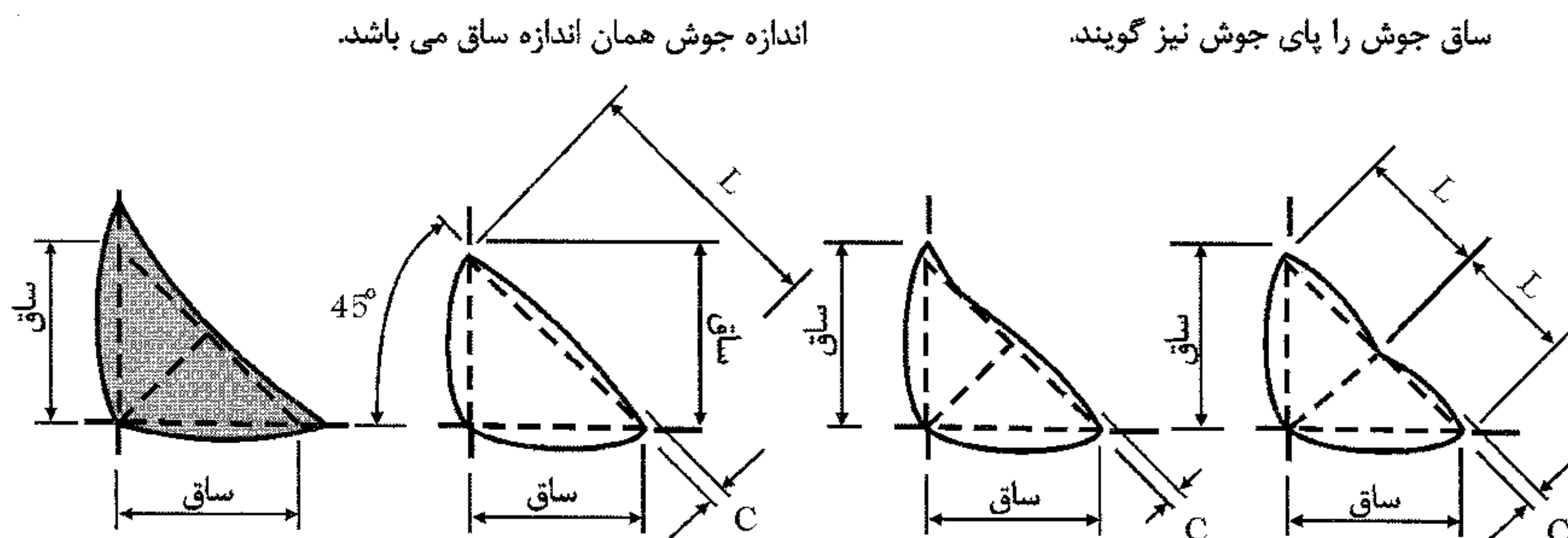
(الف) تعریف مقطع جوش گوشه
